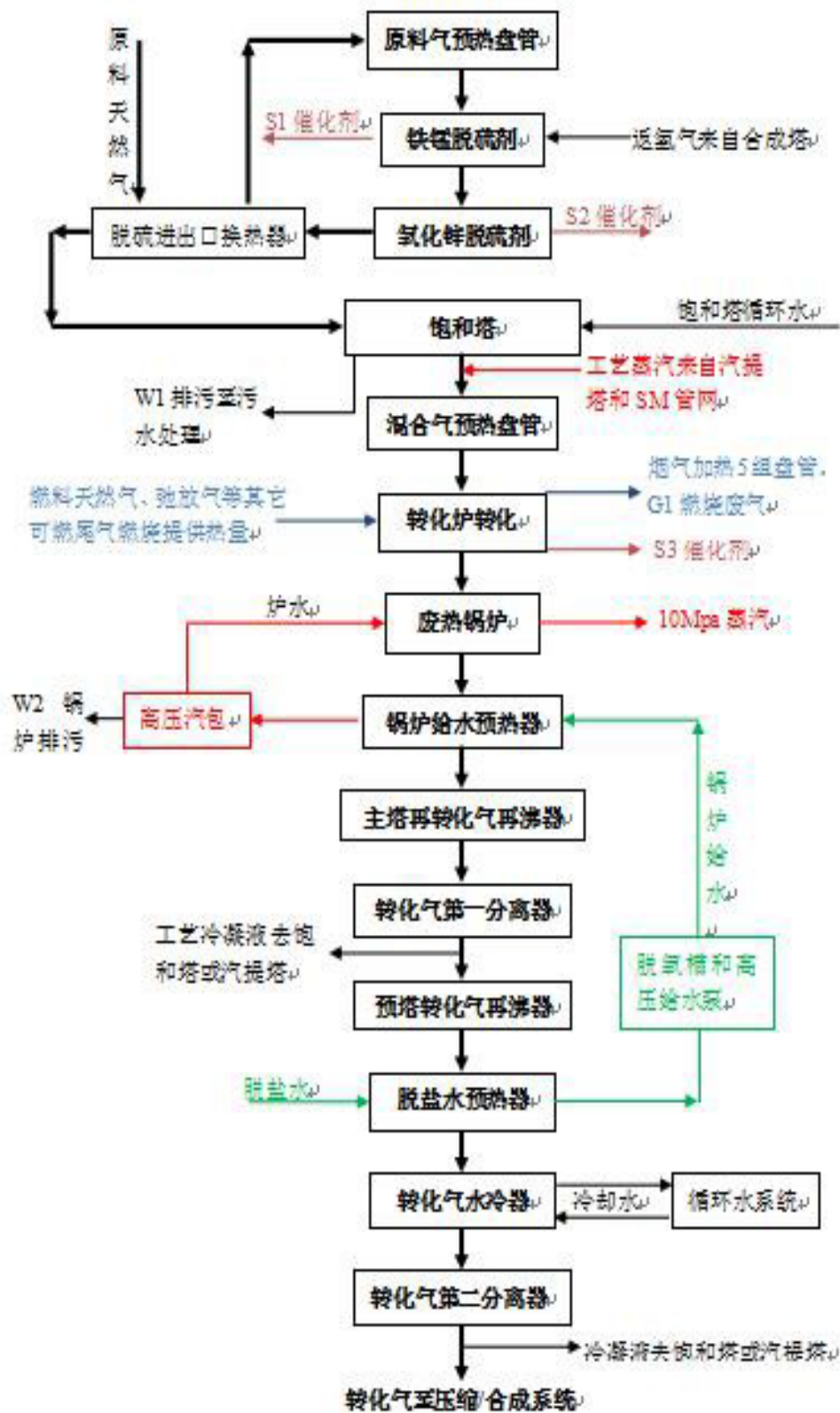
图 2-1 转化造气系统流程
