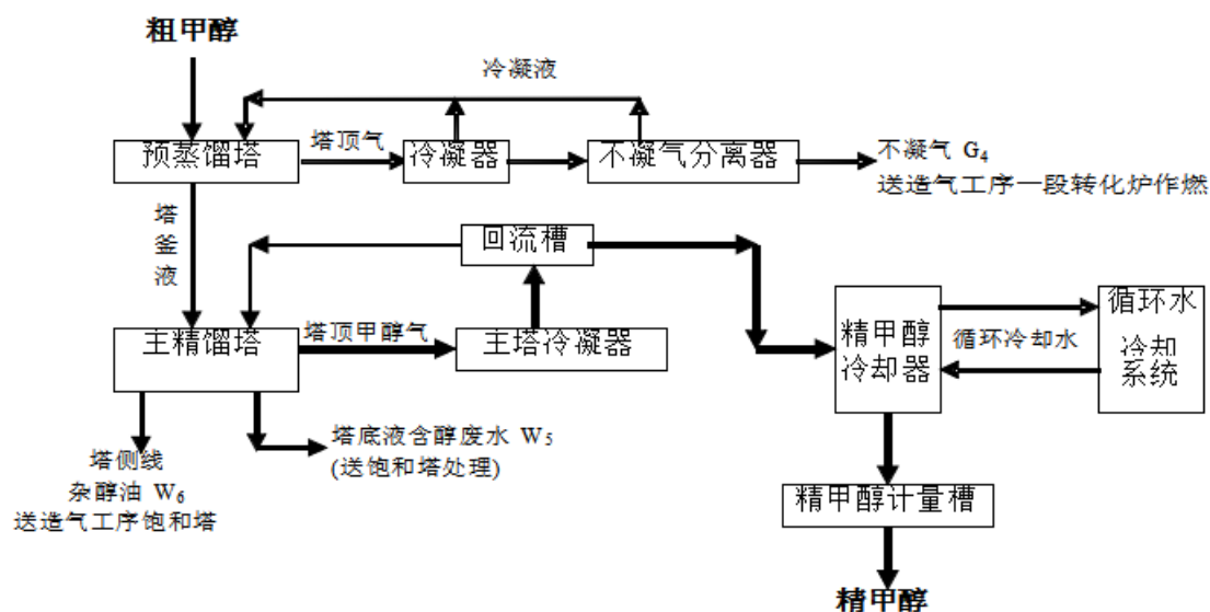
图 2-3 甲醇装置甲醇精馏工艺路程及产污位置图
